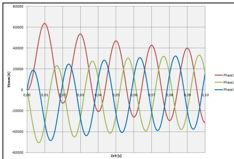
3-phasiger Kurzschlussstrom
